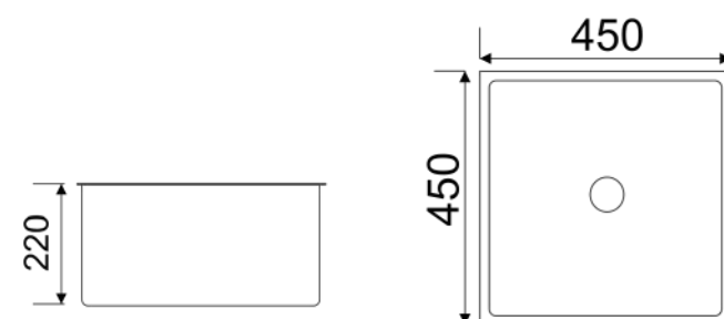
DVQ-101B-JY-120B Chậu rửa chén đơn (Đen)
