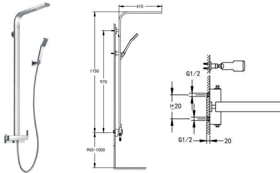
DVF-8465-1 Bộ sen cây gắn tường
