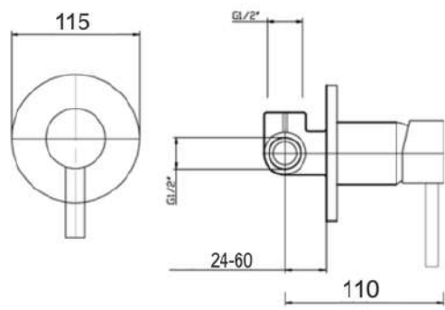
DVQ 8024 Van đóng mở 1 chức năng
