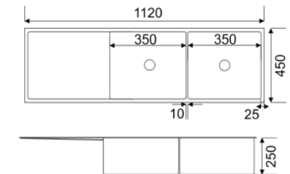
DVQ204B-JY-K121B Chậu rửa chén 2 hộc 1 cánh (Đen)
