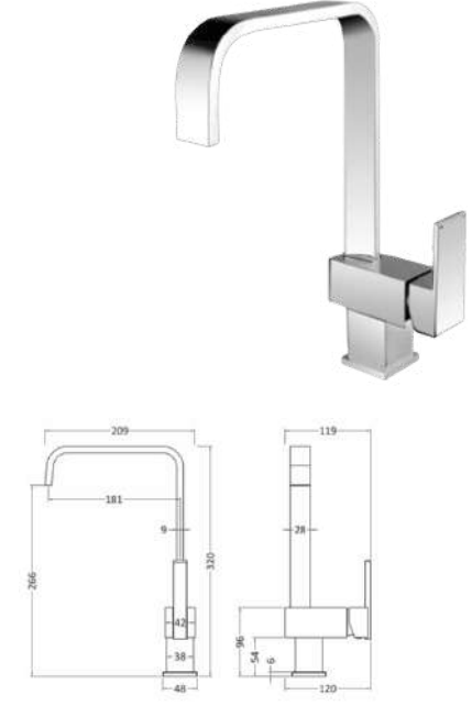
DVM 1698 Vòi bếp nóng lạnh
