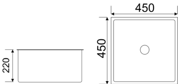
DVQ-101B-JY-120BN Chậu rửa chén đơn (Niken)
