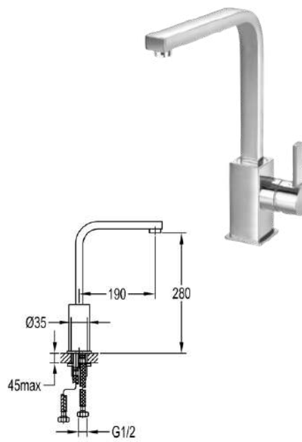
DVF-8707-2 Vòi bếp nóng lạnh
