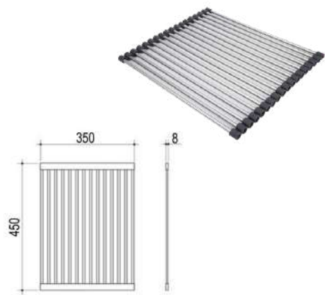
DVQ-1001 Thanh úp chén
