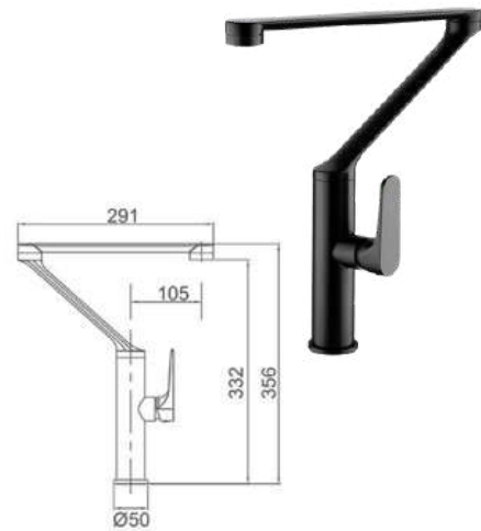
DVQ884310B Vòi bếp (màu đen)
