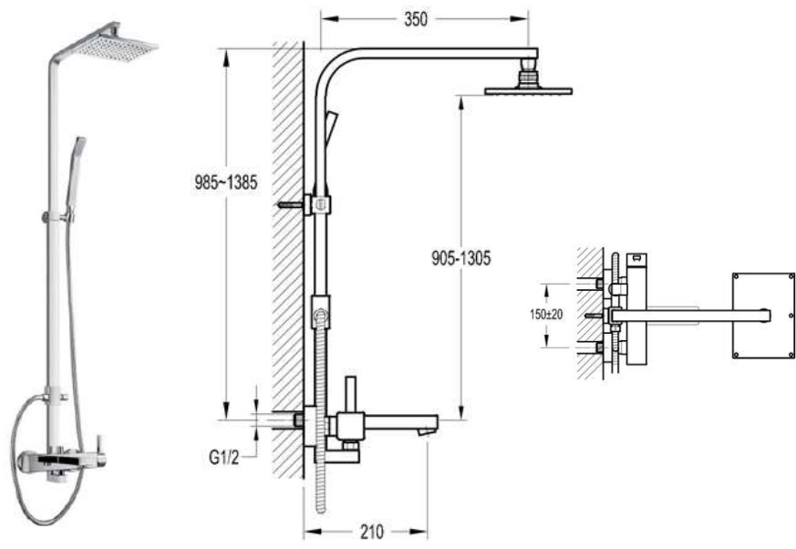
DVF-8167-1 Bộ sen cây gắn tường
