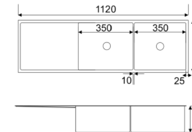
DVQ204B-JY-K121BN Chậu rửa chén 2 hộc 1 cánh (Niken)
