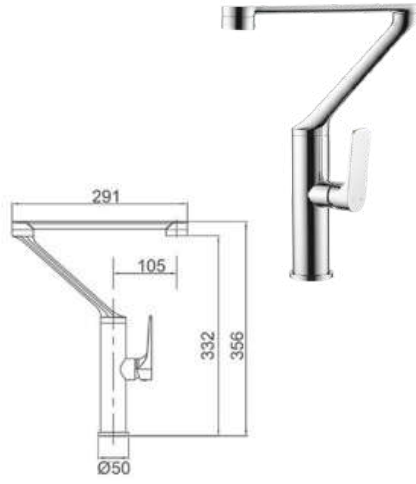
DVQ884310C Vòi bếp nóng lạnh
